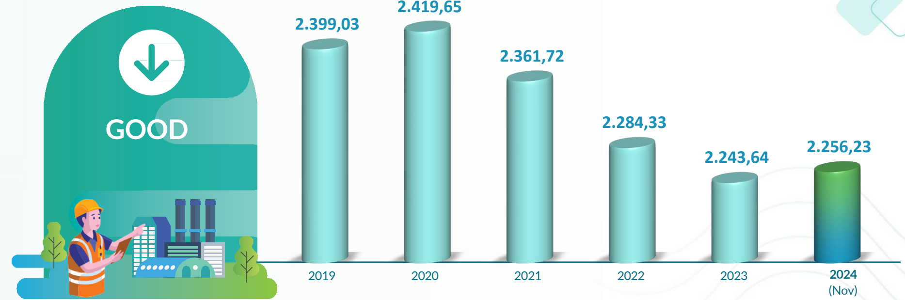
NPHR (kcal/kwh)
